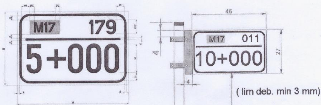
Skica 2-3 : Izgled i dimenzije znakova „kilometarska oznaka dionice magistralne ceste“ III-137
